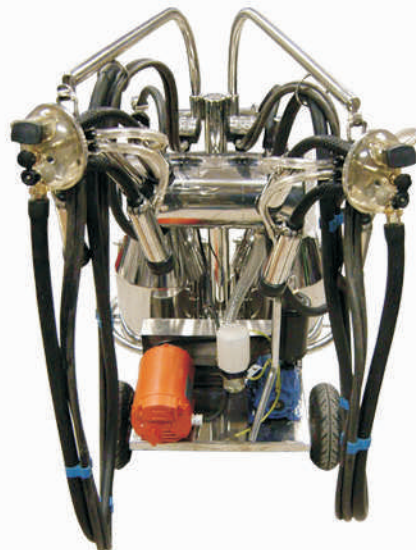
Vista Trasera
